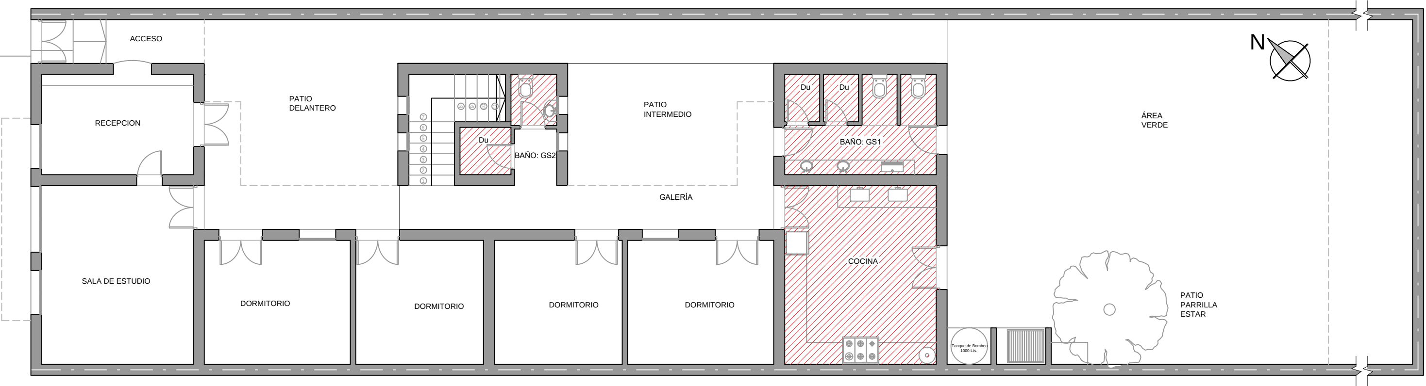
PLANTA ALTA - Esc. 1:100
