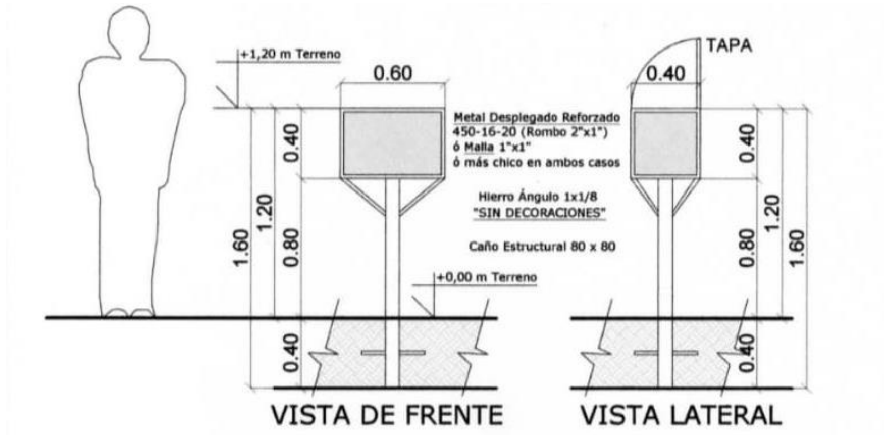
CROQUIS ESQUEMATICO (Cesto de Residuos)
