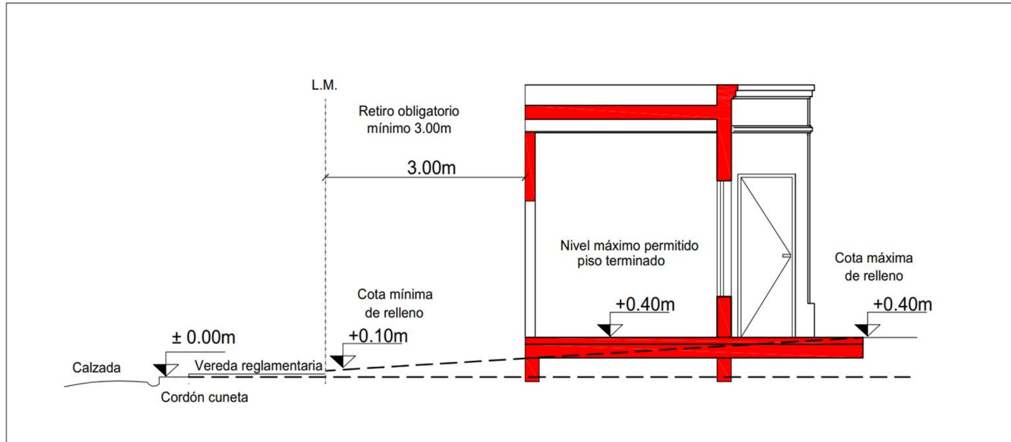
CROQUIS ESQUEMATICO (Nivelación terreno)
