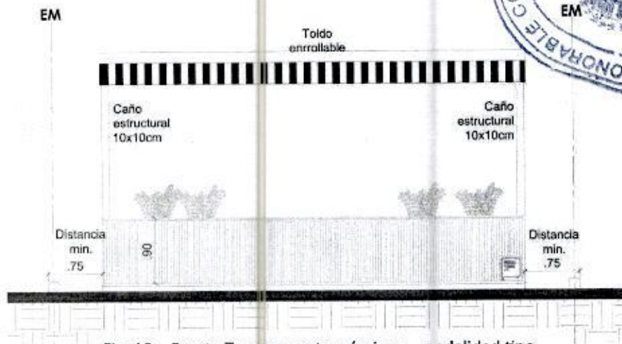
Fig. 10 - Frente Terrazas gastronómicas - modalidad tipo
