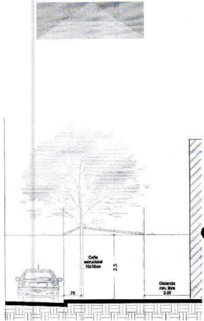
Fig. 7 - b) Toldos sobre vereda
