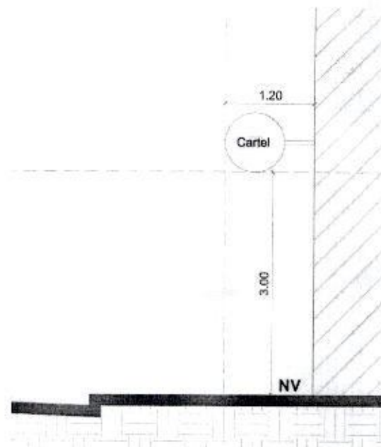
Fig. 5 - Carteles salientes sobre línea municipal
