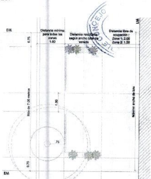
Fig. 13 - Cerramiento en vereda
