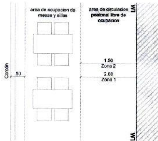
Fig. 19 – áreas de ocupación de mesas y sillas Zonas 1 y 2
