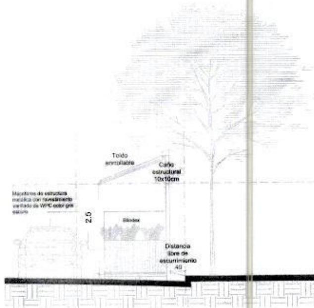
Fig. 9 - a) Corte Terrazas gastronómicas - modalidad tipo
