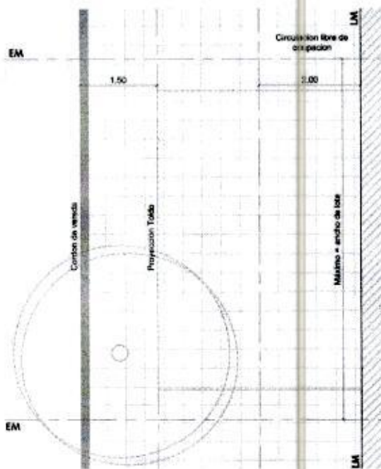
Fig. 7 - c) Planta toldos sobre fachadas
