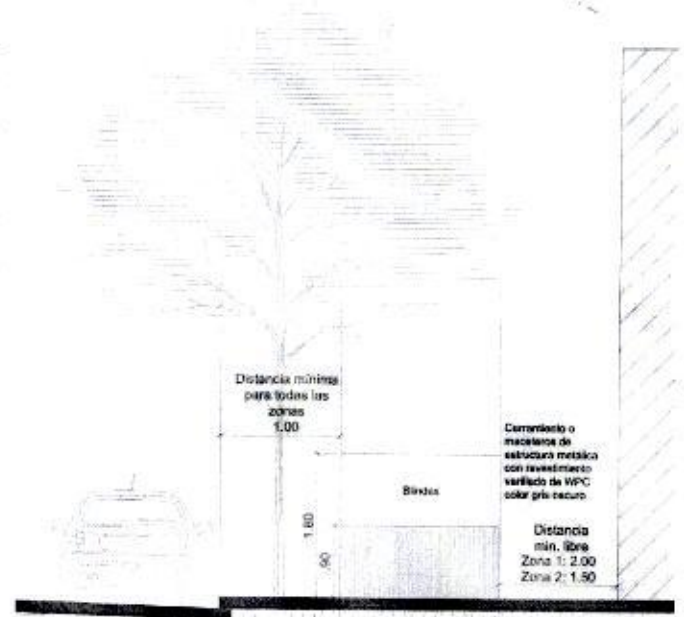
Fig. 15 – Vista cerramiento en veredas
