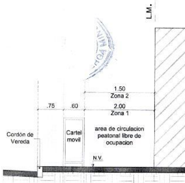
Fig. 3 - Carteles o pizarras en veredas
