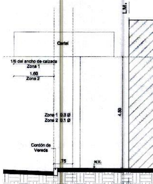
Fig. 5 – Carteles salientes sobre calzadas
