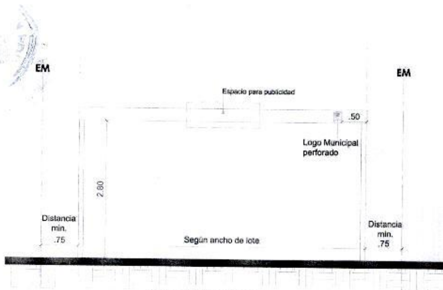
Fig. 8- d) Frente Aleros
