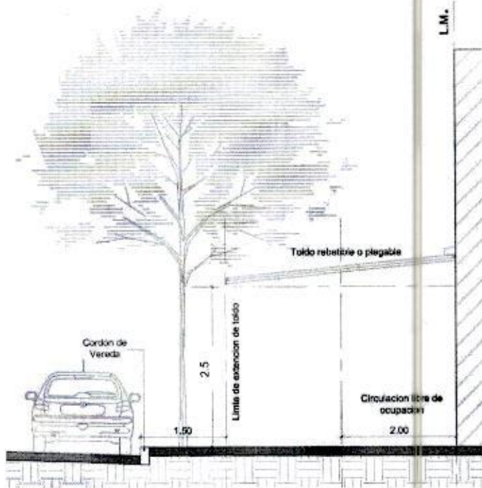
Fig. 7 - a) Toldos sobre fachadas
