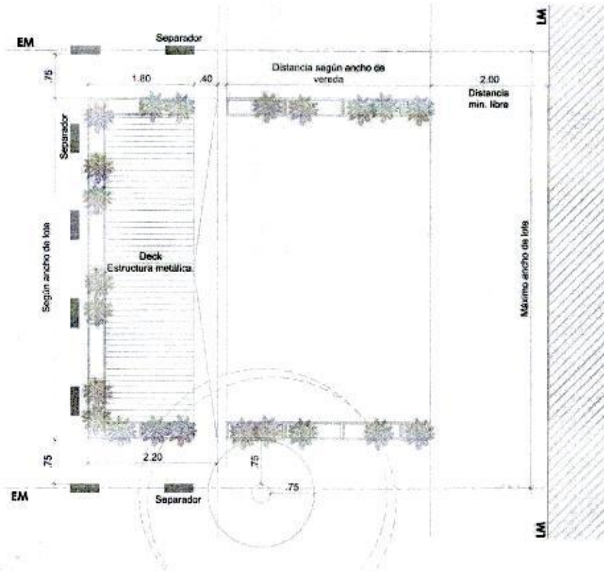
Fig. 11 – Terrazas gastronómicas y cerramiento en vereda
