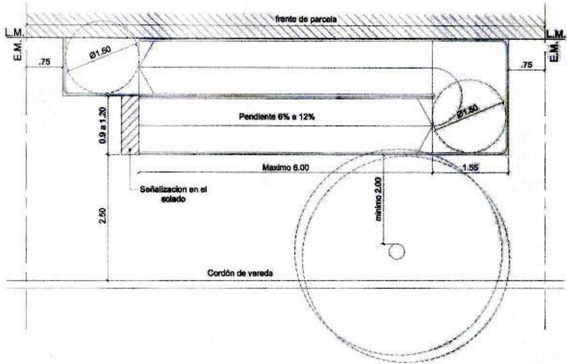
Fig. 22 – Rampas en veredas (excepcionalmente y únicamente en Zona 1)
