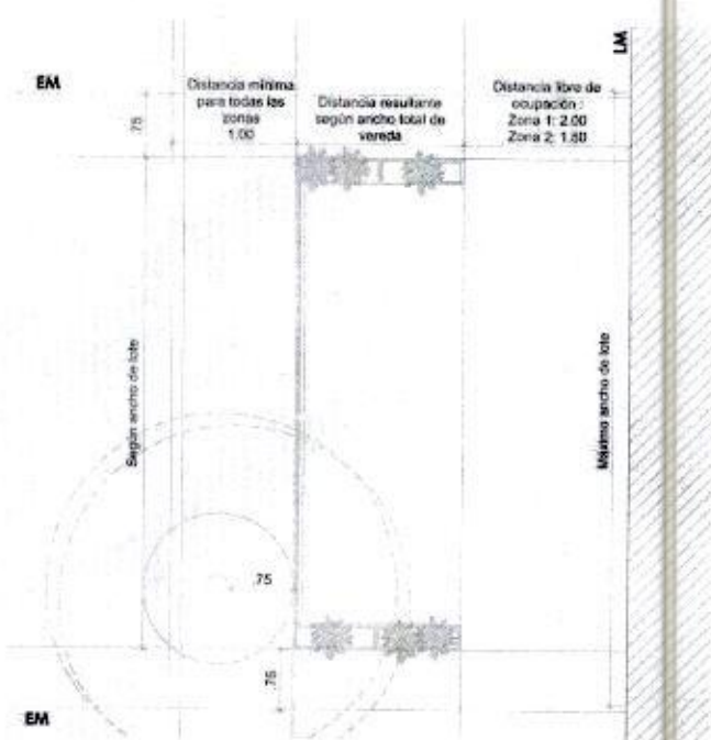
Fig. 12 - Cerramiento en vereda
