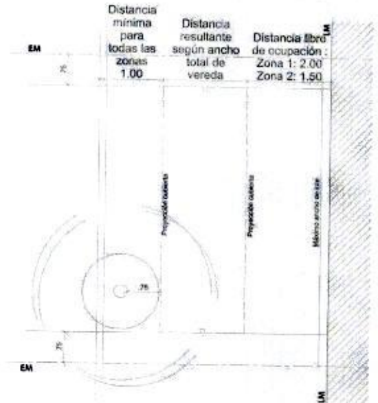
Fig. 8- c) Planta Aleros con un apoyo
