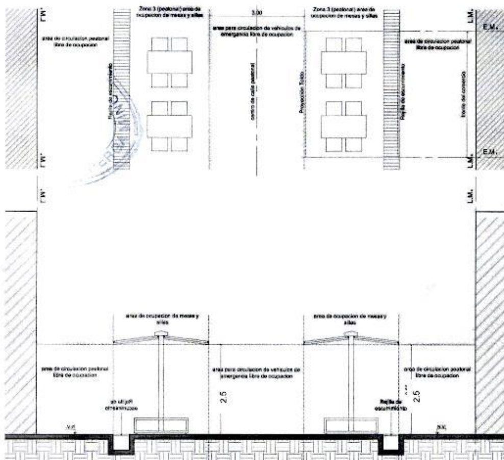
Fig. 20 – áreas de ocupación de mesas y sillas Zonas 3 – Peatonal San Nicolás
