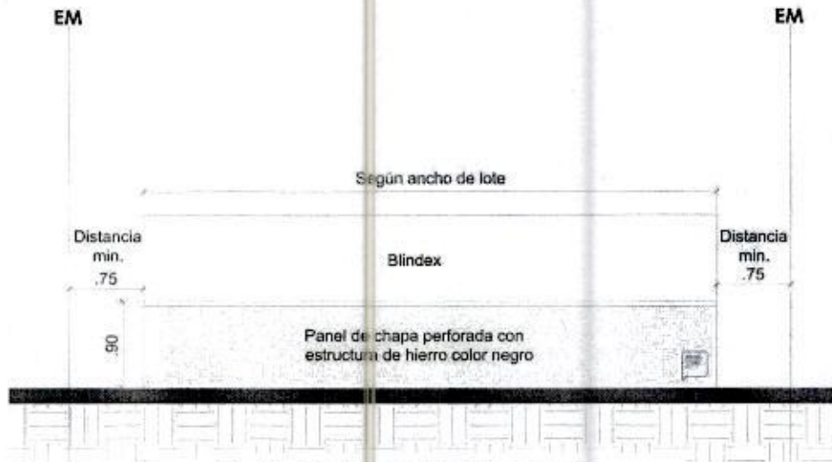
Fig. 17 – Frente cerramiento en veredas
